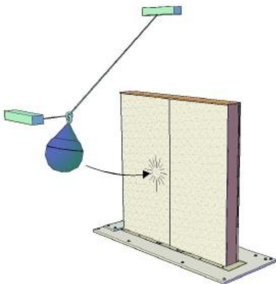
Figure 1 : Schéma de principe de l'essai avec le choc mou « M50 »
